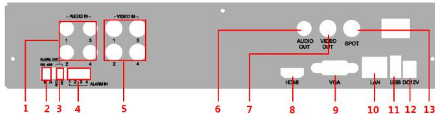
Задняя панель 4-канального прибора
