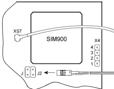
Рисунок 14.3 – Коммуникатор и термодатчик
