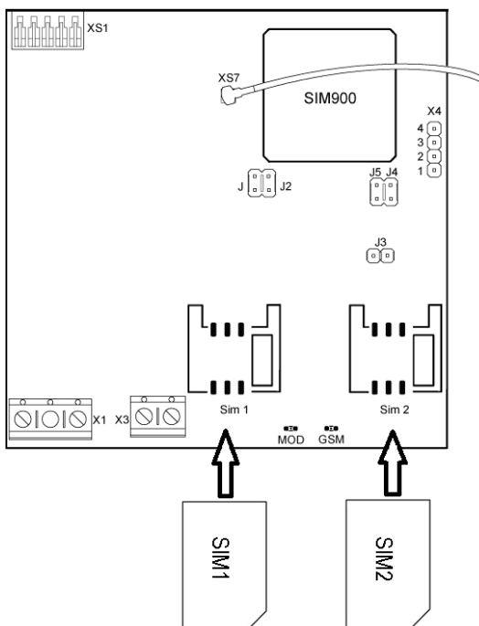
Рисунок 14.1 – Коммуникатор
