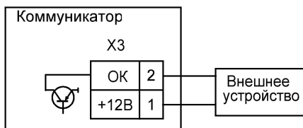
Рисунок 14.2 – Схема подключения внешнего устройства к коммуникатору
